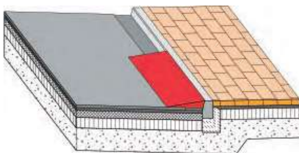
Рисунок 59– Пример обустройства короткого пандуса на временном пешеходном пути
