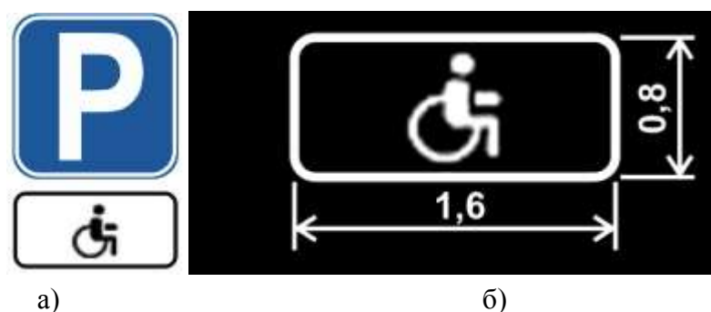
Рисунок 55 – Пример обозначения машино-места для стоянки (парковки) транспортного средства инвалидов с использованием дорожных знаков (а) и дорожной разметки (б)
