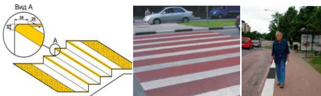
Рисунок 72– Примеры выполнения контрастных покрытий
