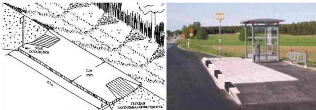
Рисунок 48– Пример обустройства остановочного пункта пандусами
