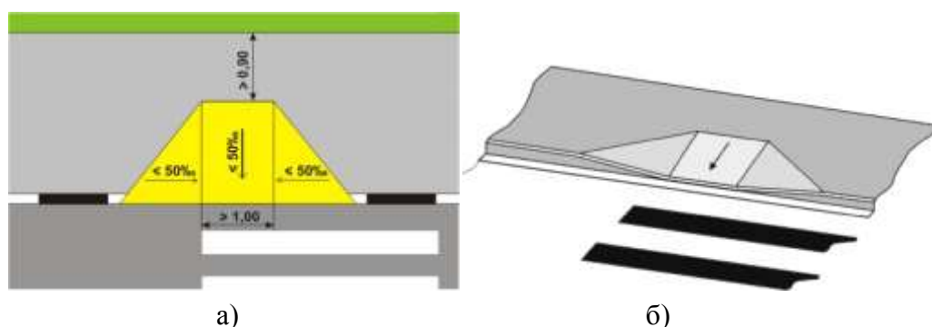
Рисунок 29– Вариант размещения пандусов на отнесенных пешеходных переходах и пешеходных переходах, располагаемых на перегонах
