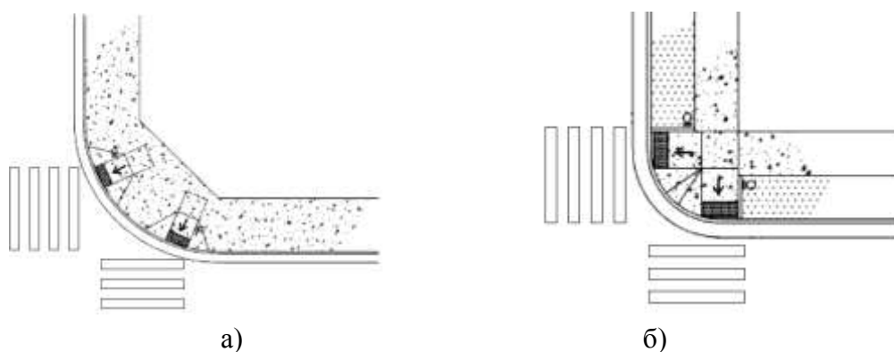
Рисунок 30– Варианты размещения пандусов на пешеходных переходах, выполненных по продолжению тротуара (пешеходной дорожки)
