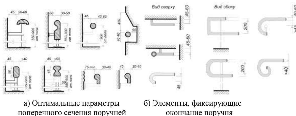
Рисунок 13 – Основные параметры конструкции поручней
