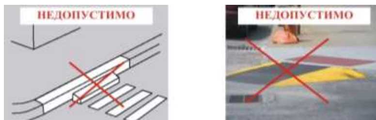
Рисунок 35 – Примеры неправильного выполнения пандусов на пешеходных переходах
