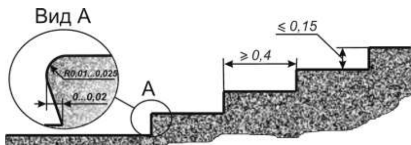
Рисунок 9– Основные параметры ступеней
