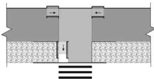
Рисунок 34 – Пример поэтапного понижения уровня тротуара перед пешеходным переходом
