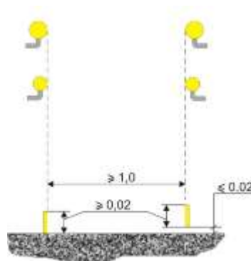
Рисунок 14– Параметры размещения бортиков безопасности
