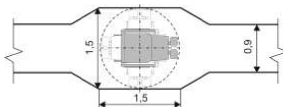
Рисунок 6 – Пример выполнения зоны изменения направления движения людей в кресле-коляске для стесненных условий
