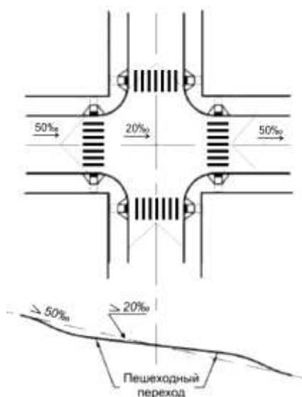
Рисунок 19 – Схема приподнятой зоны перекрестка
