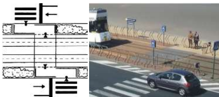
Рисунок 43 – Пример размещения пешеходного перехода через трамвайные пути
