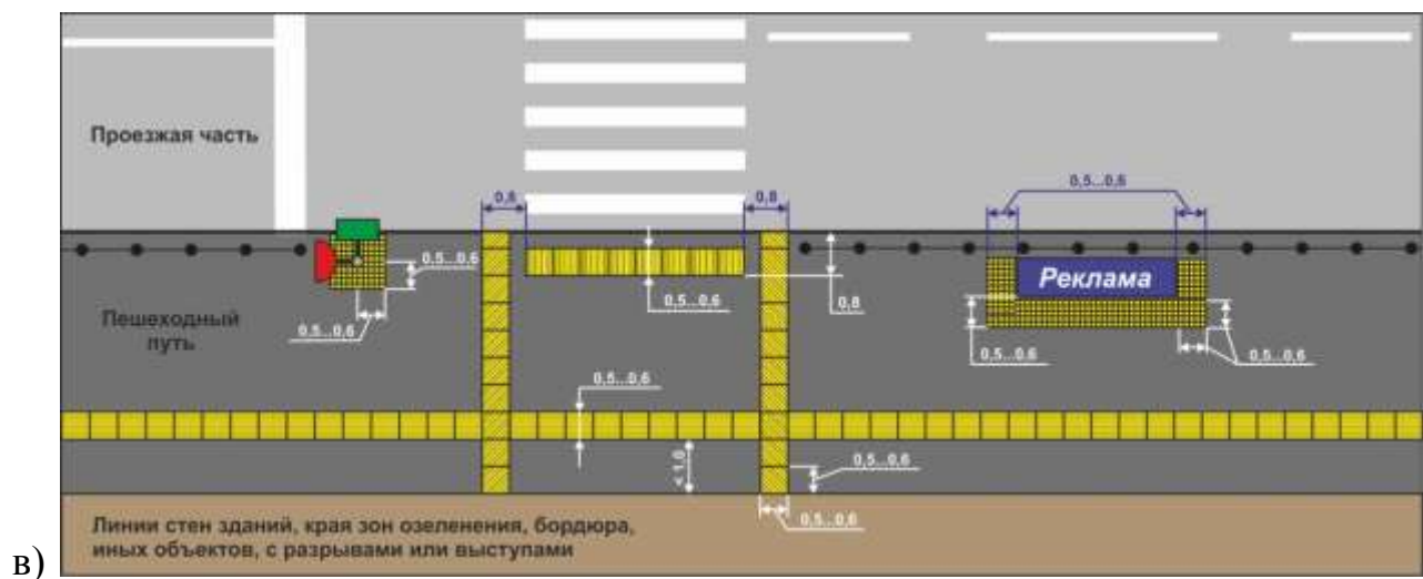
Рисунок Г.3 – Типовые схемы обустройства пешеходных путей и пешеходных переходов тактильными наземными указателями:
