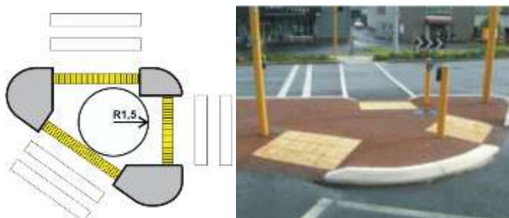
Рисунок 36 – Пример обеспечения доступности островка безопасности для людей в кресле-коляске и других маломобильных групп населения
