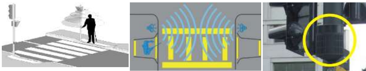
Рисунок 71 – Примеры размещения направленности действия технических средств звуковой сигнализации на регулируемых пешеходных переходах
