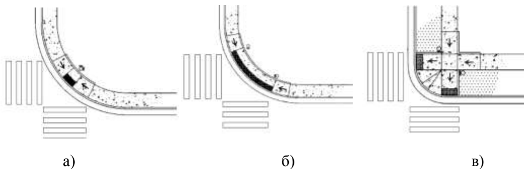
Рисунок 32– Варианты размещения пандусов на пешеходных переходах, выполненных по продолжению тротуара (пешеходной дорожки) в стесненных условиях
