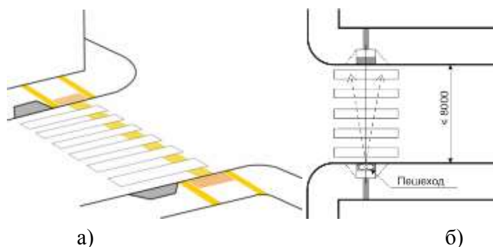
Рисунок 64 – Примеры обустройства пешеходных переходов тактильной направляющей поверхностью
