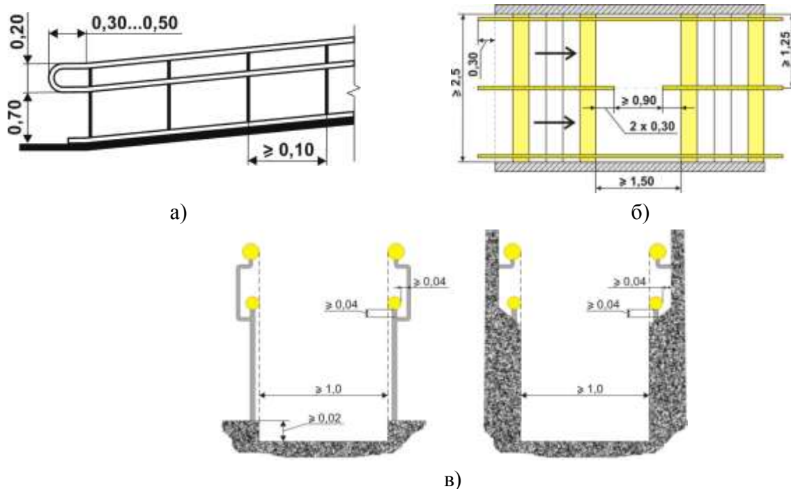
Рисунок 12– Основные параметры размещения перил и поручней в пределах лестниц и пандусов
