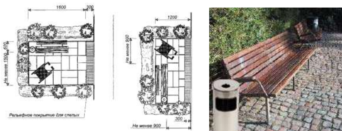
Рисунок 56 – Примеры обустройства зон отдыха инвалидов
