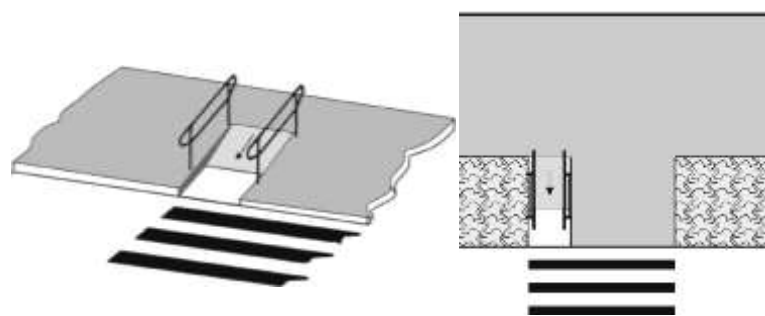
Рисунок 25– Вариант размещения пандусов на отнесенных пешеходных переходах и пешеходных переходах, располагаемых на перегонах
