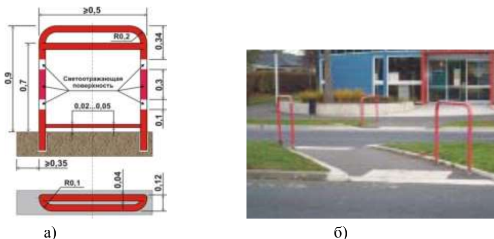
Рисунок 38– Рекомендуемая форма конструкции и основные параметры пешеходного ограждения (а), пример применения (б)
