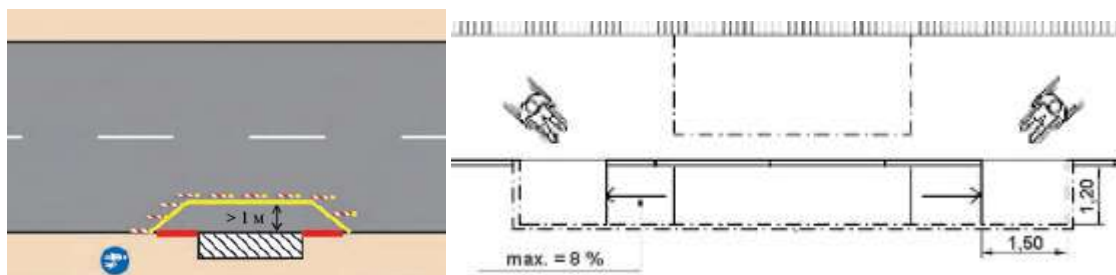
Рисунок 58– Примеры обустройства временного пешеходного пути
