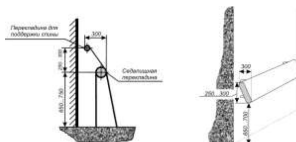
Рисунок В.7 – Основные параметры конструкции скамьи наклонного типа
